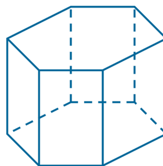
graniastosłup prosty sześciokątny
